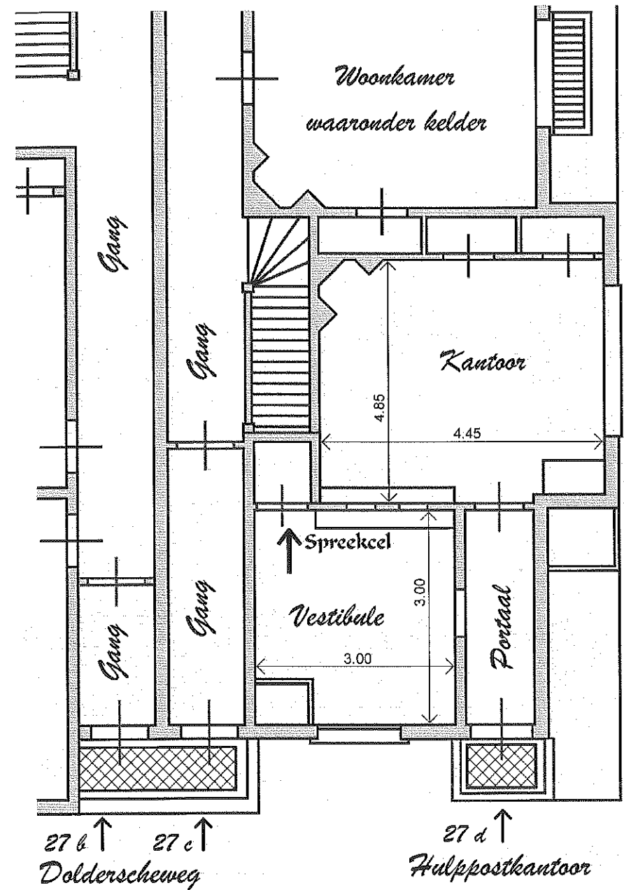
Bouwtekening hulppostkantoor Dolderseweg 27a (115)
