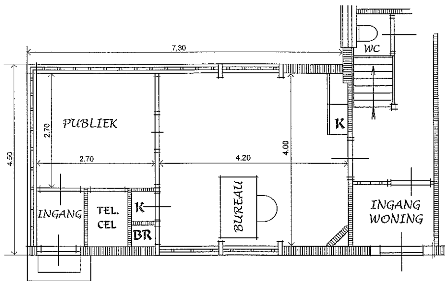
Bouwtekening postkantoor Dolderseweg 112.
