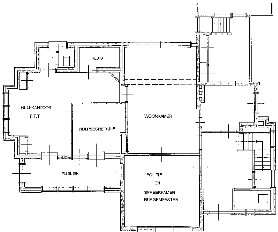
Bouwtekening van het pand Dolderseweg 71 (tekening uit 1951)
